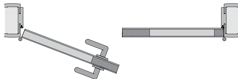
БГ Ляв нормал EN Left portal IT Portale sinistra
